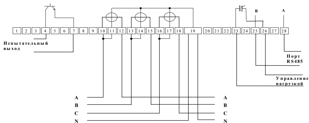
Рисунок В.1 – Схема подключения счетчика непосредственного включения
