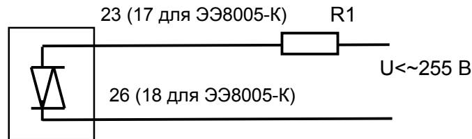
Рисунок 4.2 - Схема подключения выхода устройства управления нагрузкой
