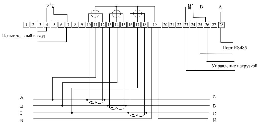
Рисунок В.2 – Схема подключения счетчика трансформаторного включения
